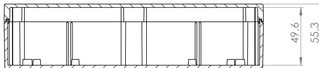
PRZEKRÓJ J-J
