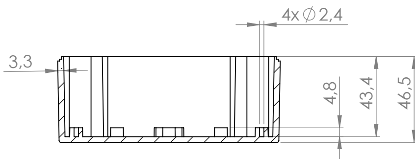
PRZEKRÓJ B-B
