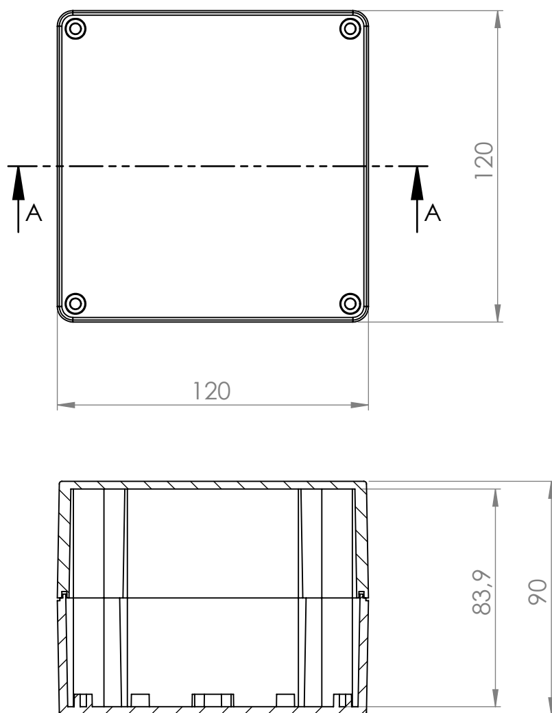
PRZEKRÓJ A-A
