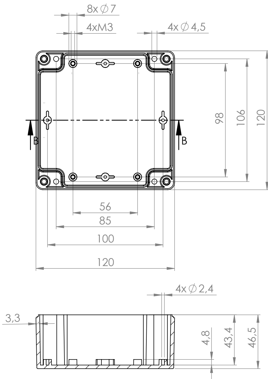
PRZEKRÓJ B-B
