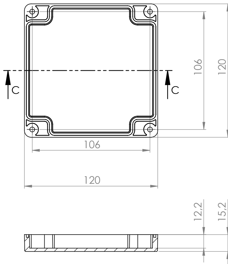
PRZEKRÓJ C-C
