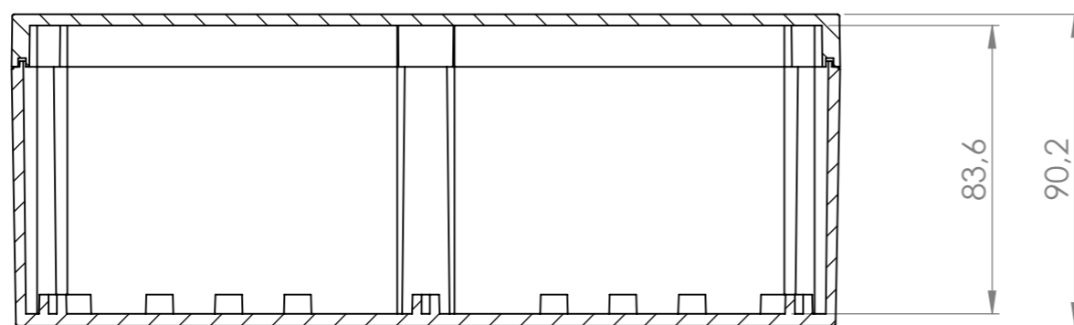
PRZEKRÓJ A-A
