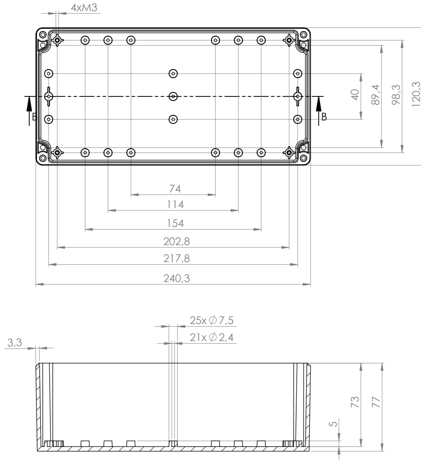
PRZEKRÓJ B-B
