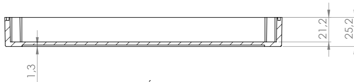
PRZEKRÓJ C-C
