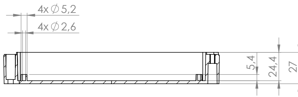
PRZEKRÓJ B-B
